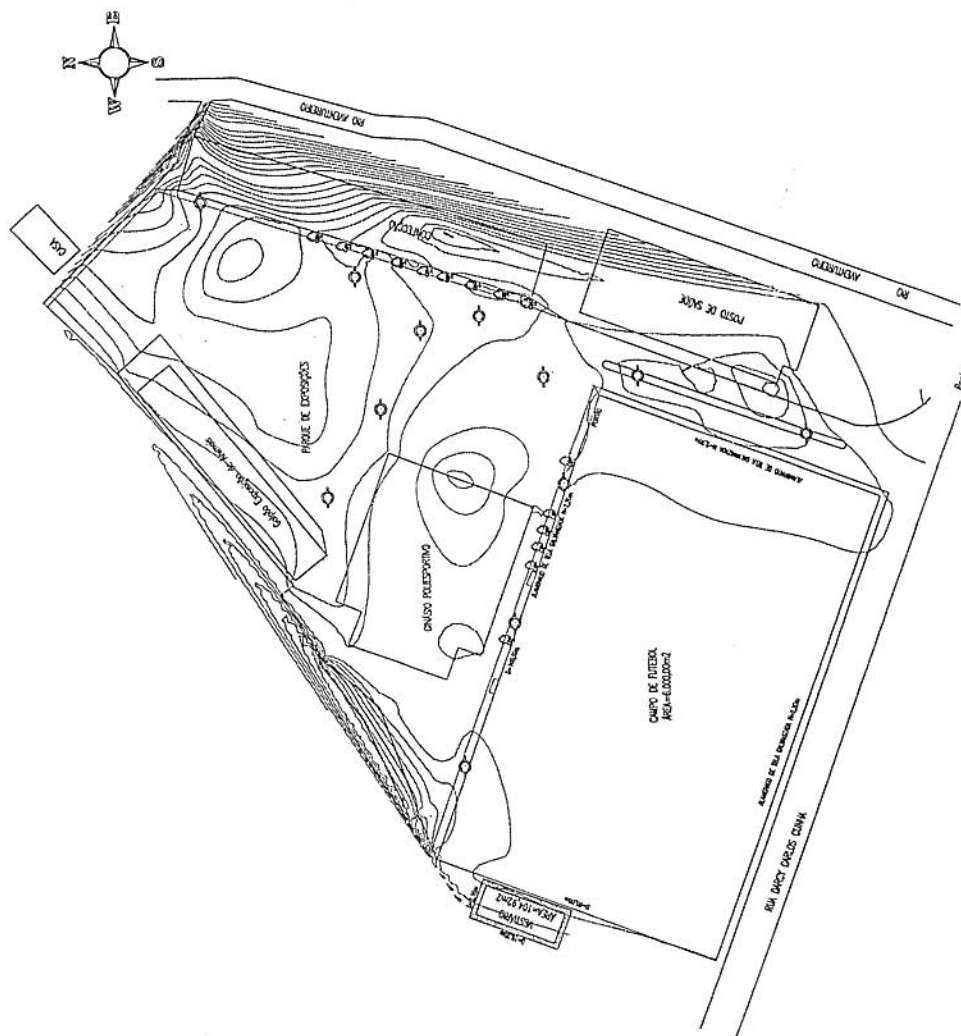
1. LEVANTAMENTO PLANIMÉTRICO Escala 1:500
