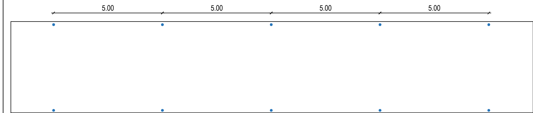
1 DRENAGEM Escala 1:250
