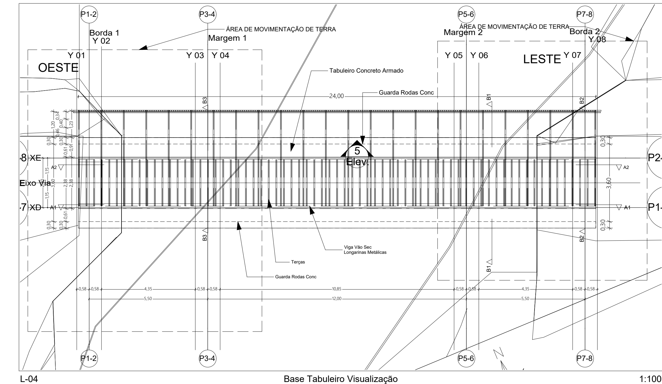
L-04 Base Tabuleiro Visualização 1:100
