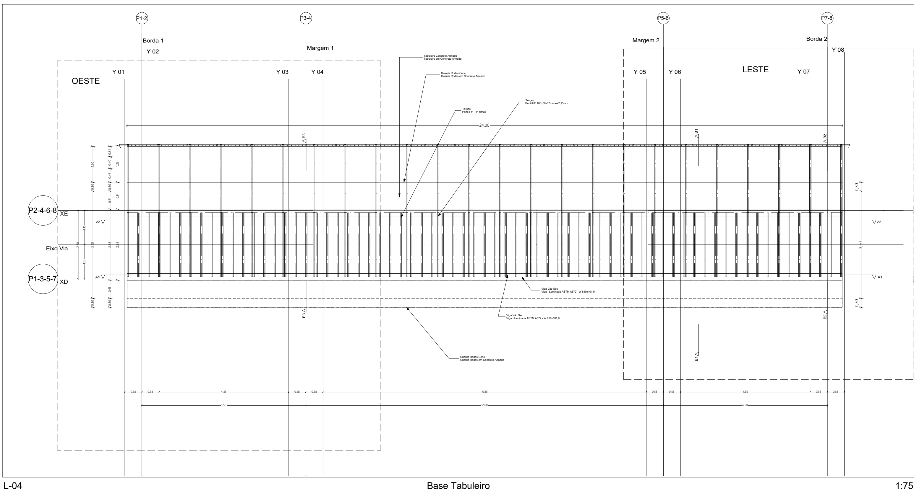
L-04 Base Tabuleiro 1:75
