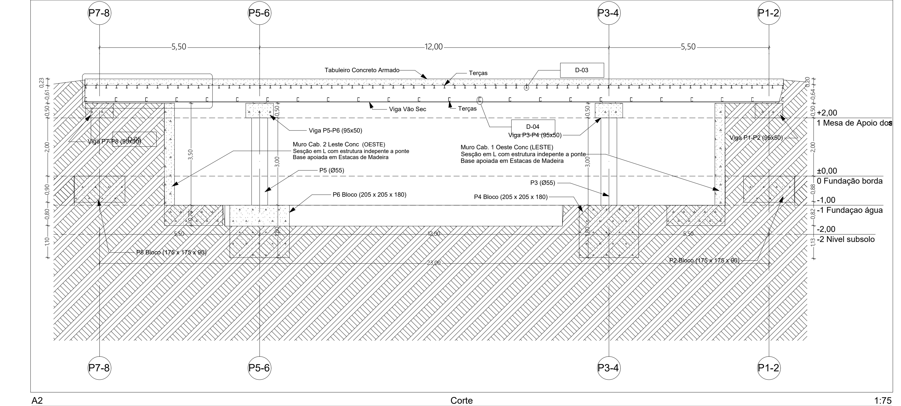
A2 Corte 1:75
