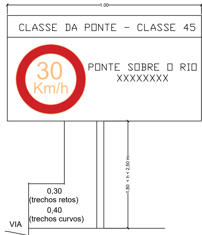
2 DETALHE DE PLACA SEM ESCALA
