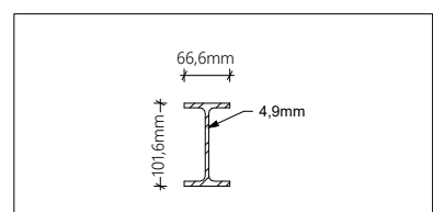
D-03 Perfil I Terças 1:10
