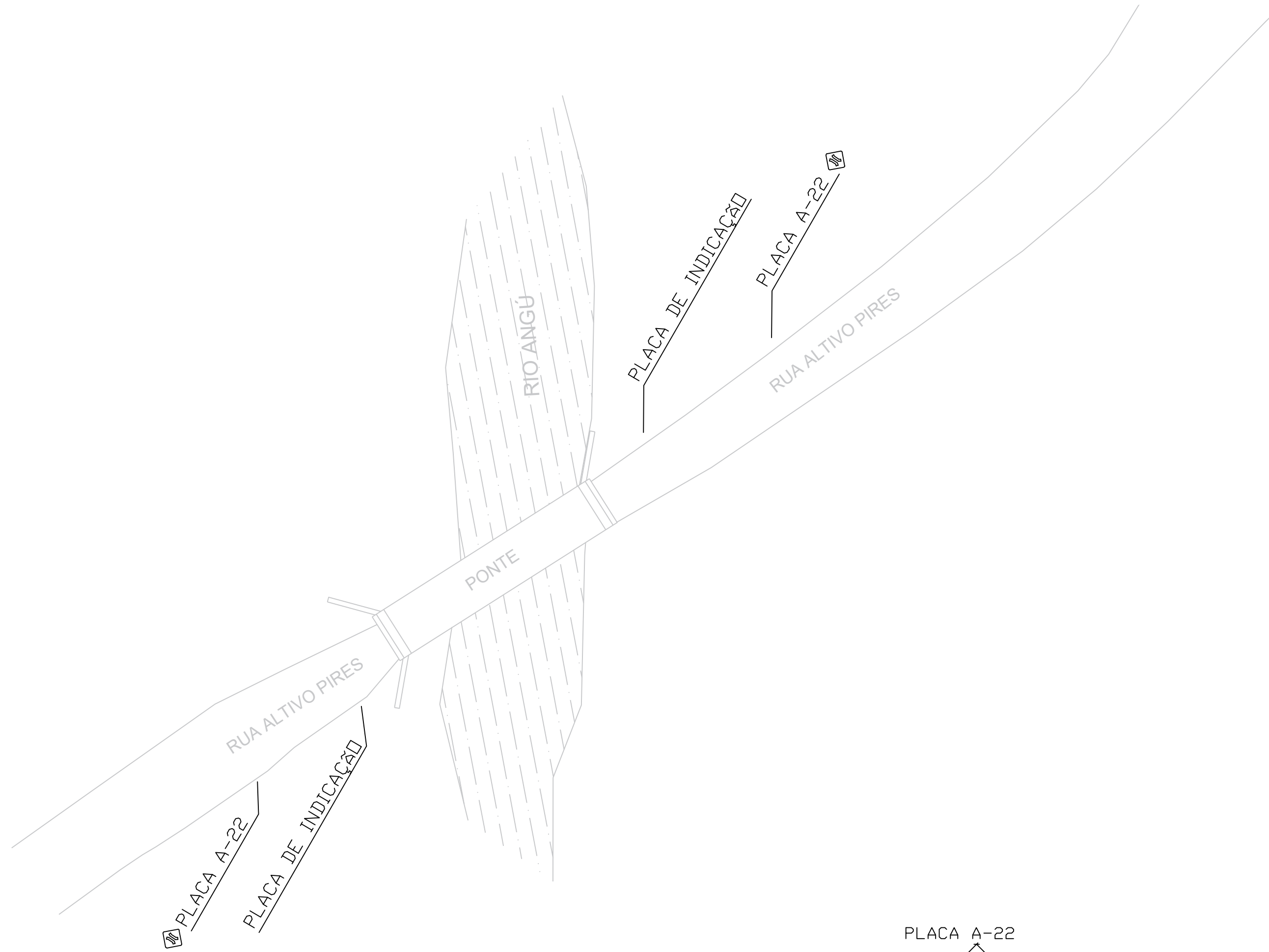
1 SINALIZAÇÃO Escala 1:300
