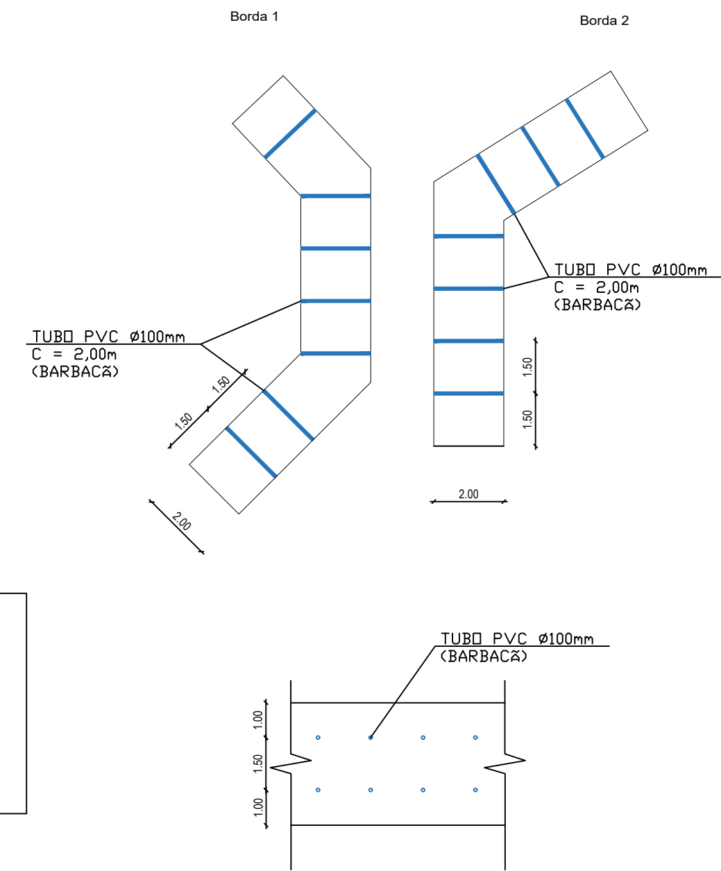
3 DETALHES DA DRENAGEM DO MURO - BARBACÃ ESCALA 1:150
