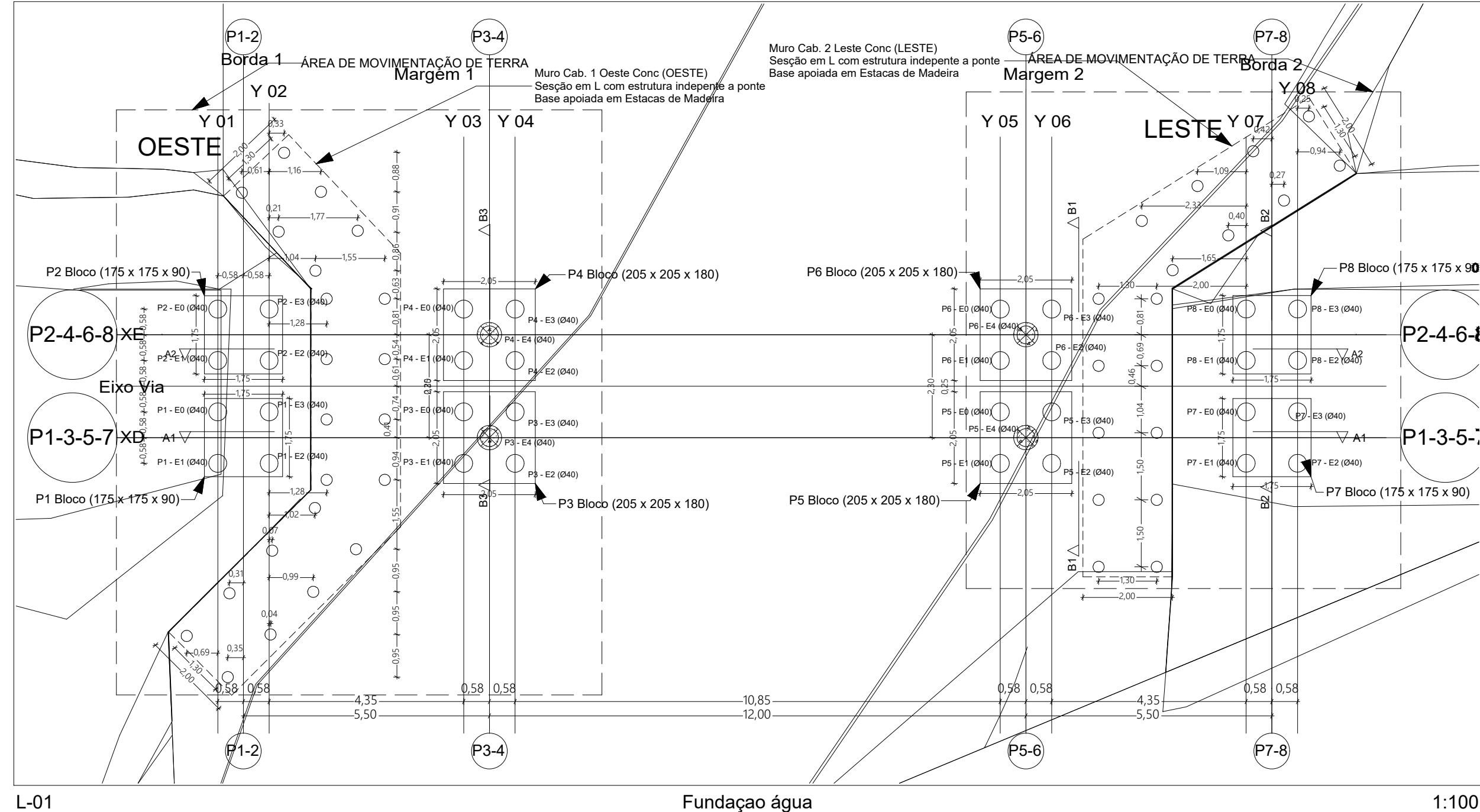
L-01 Fundação água 1:100
