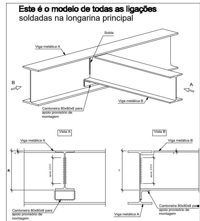
D-07 Solda de Vigas na Longarina
