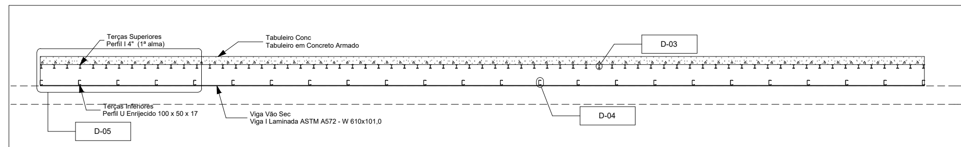
A2 Corte Posição Terças 1:100
