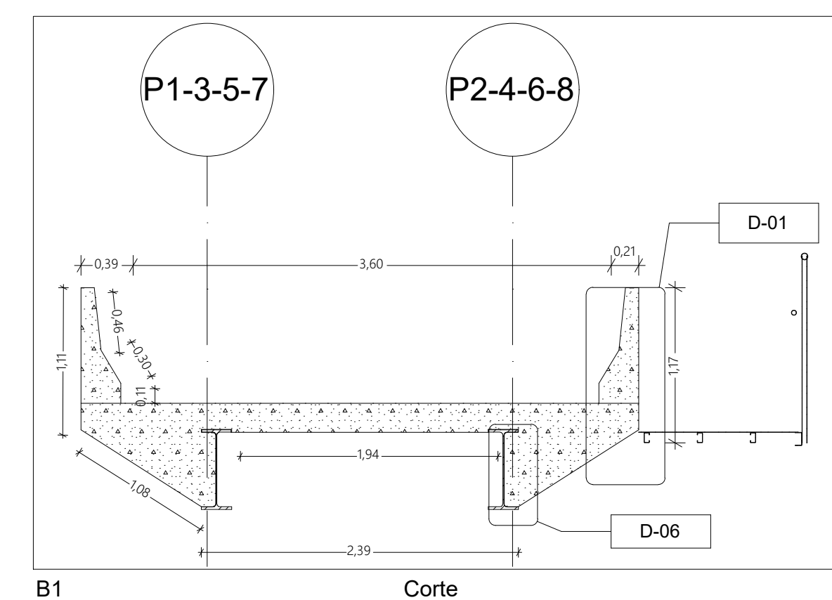
B1 Corte
