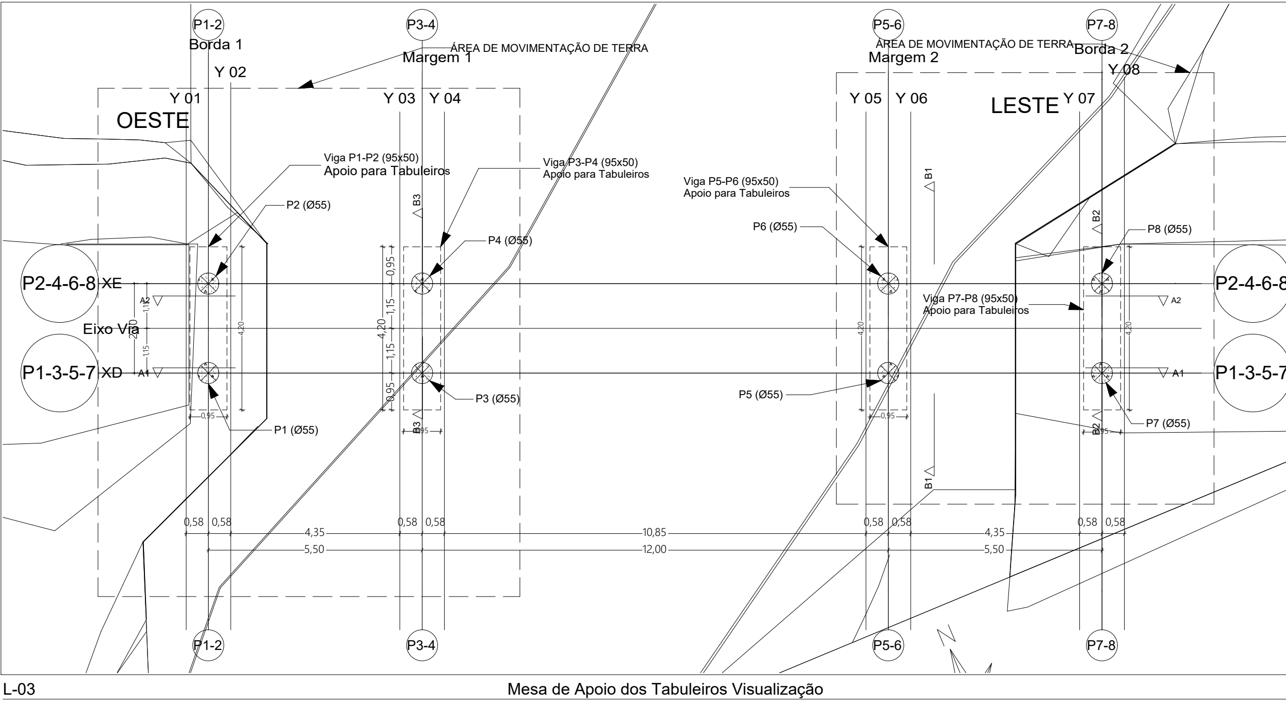
L-03 Mesa de Apoio dos Tabuleiros Visualização 1:100
