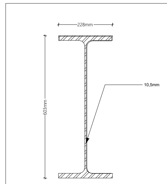
D-06 Viga Principal 1:10
