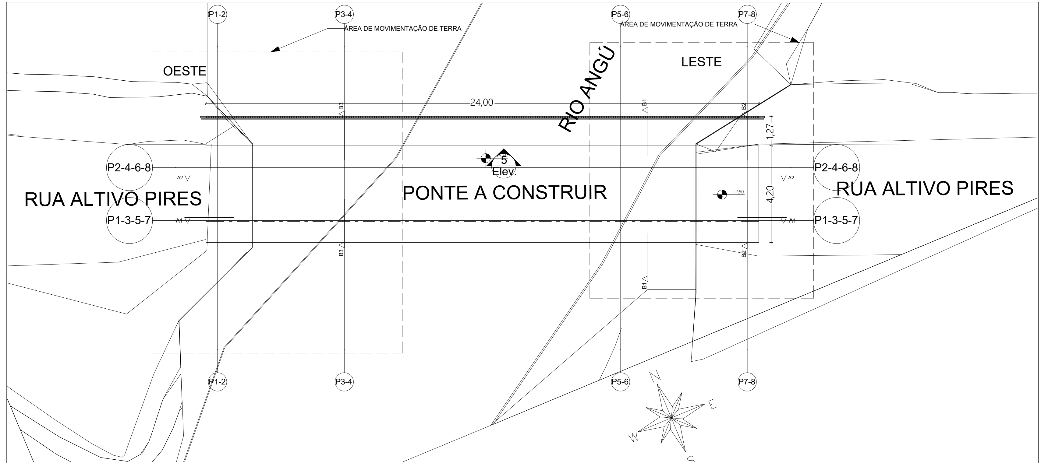
L-05 Vista Implantação Sobreposta com Arquitetura 1:100
