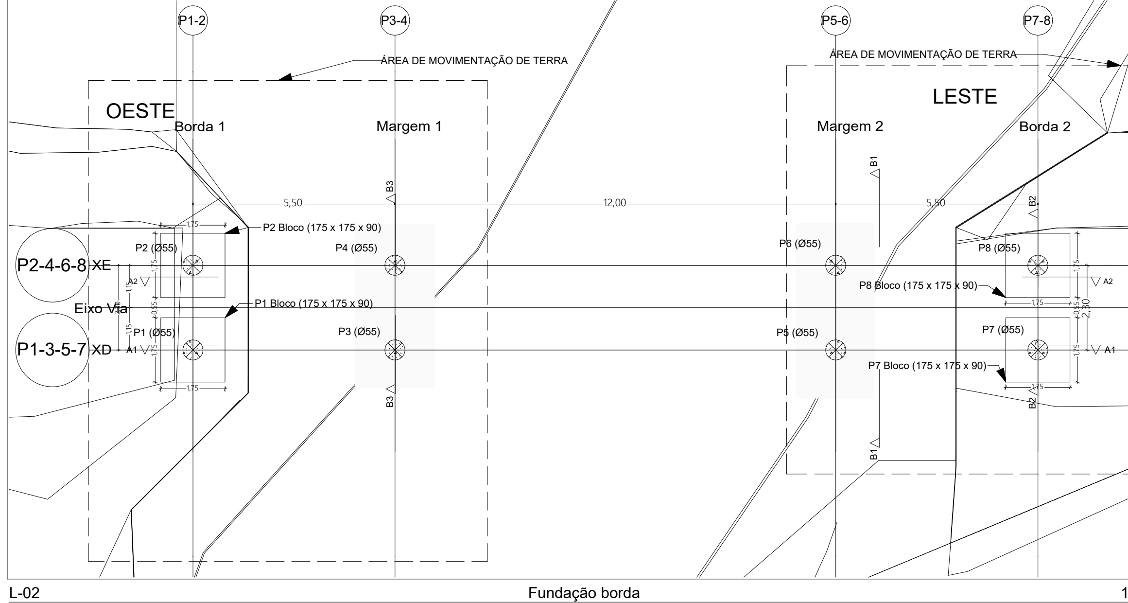
L-02 Fundação borda 1:100
