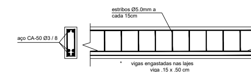
3 DETALHES PASSAGEM ELEVADA Escala 1:100
