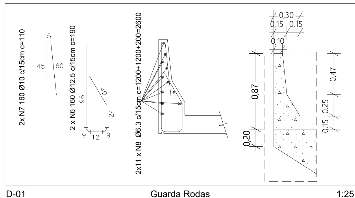
D-01 Guarda Rodas 1:25
