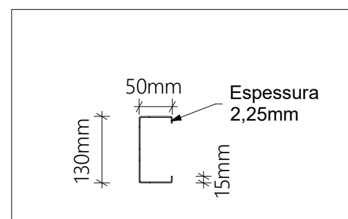
D-04 Perfil U Enrijecido 1:10
