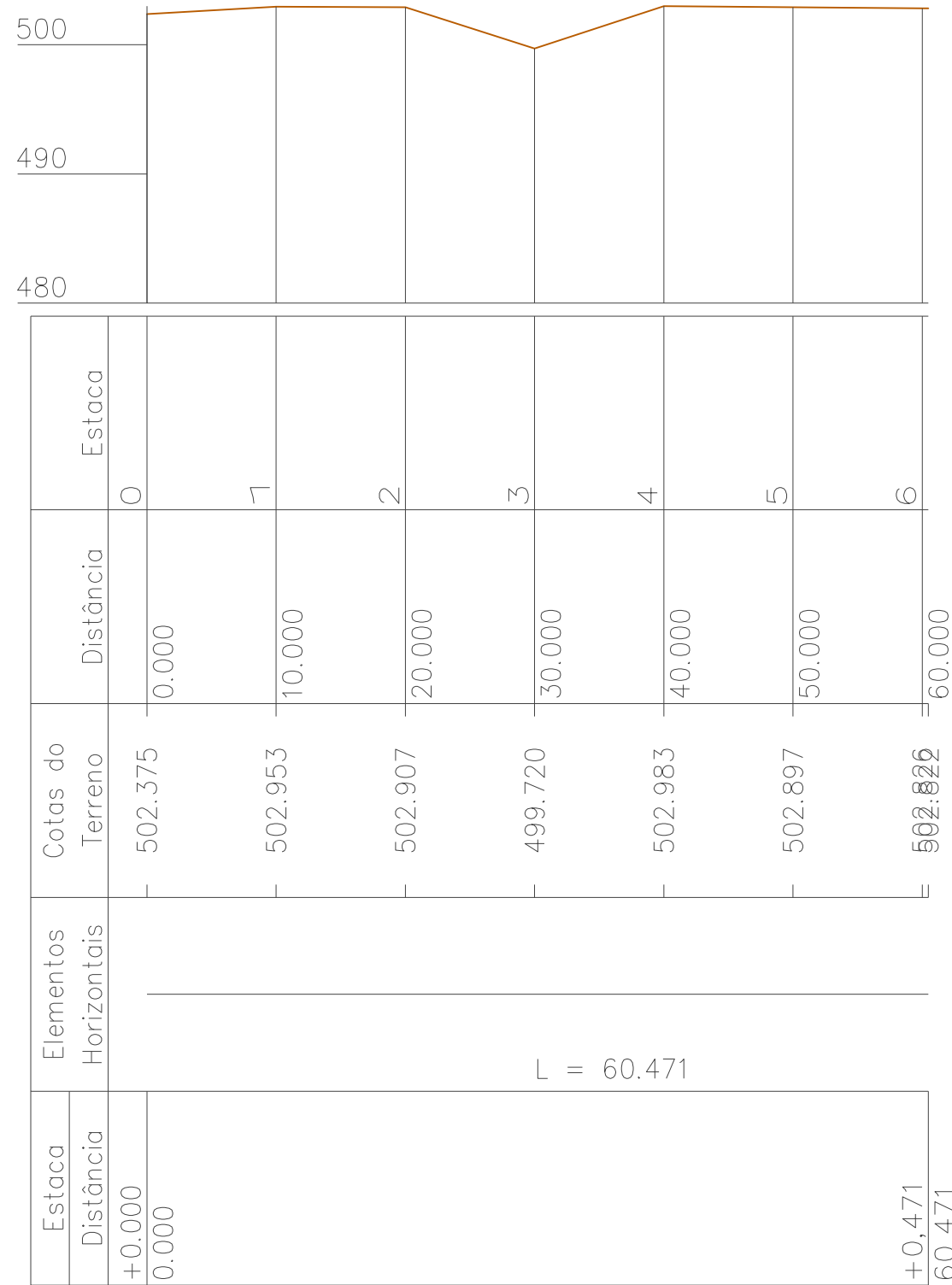
3 PERFIL ESCALA 1:500
