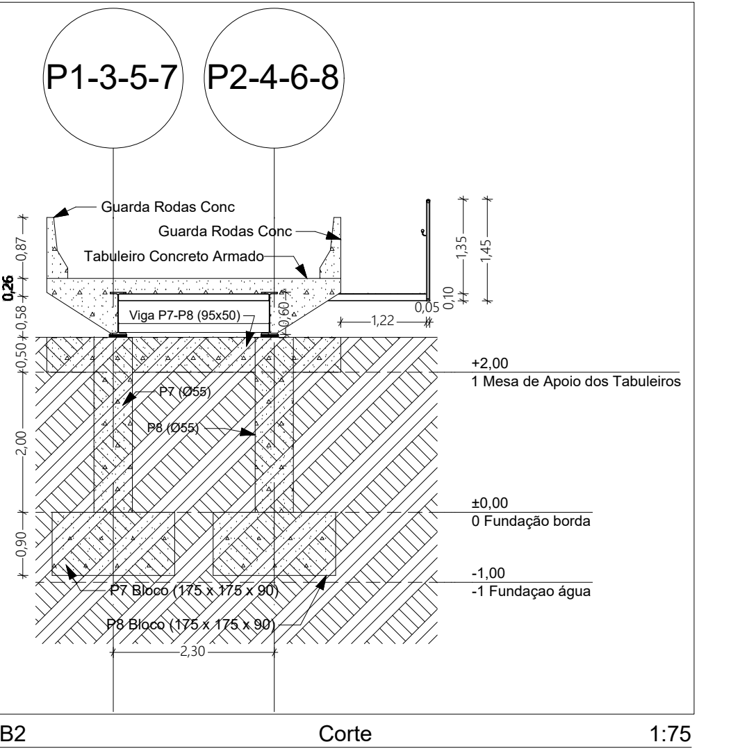
B2 Corte 1:75
