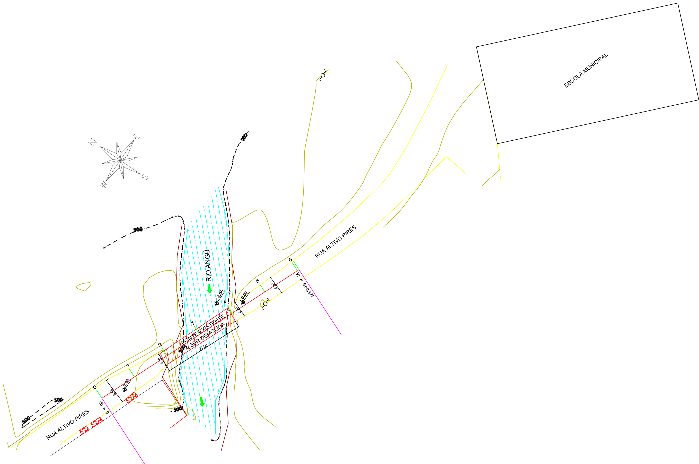
1 LEV. TOPOGRÁFICO PLANIALTIMÉTRICO Escala 1:500
