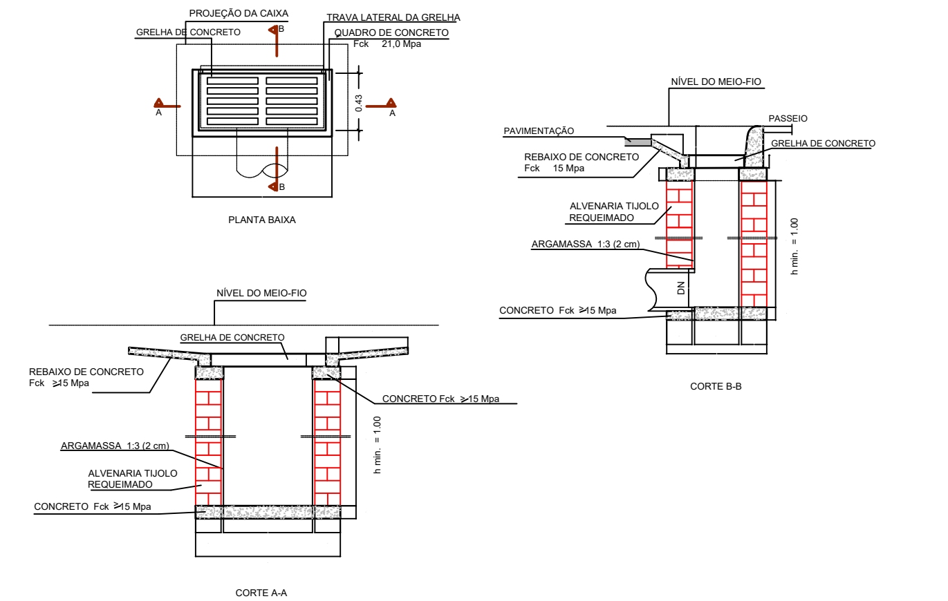
2 DETALHES DA BOCA DE LOBO SEM ESCALA
