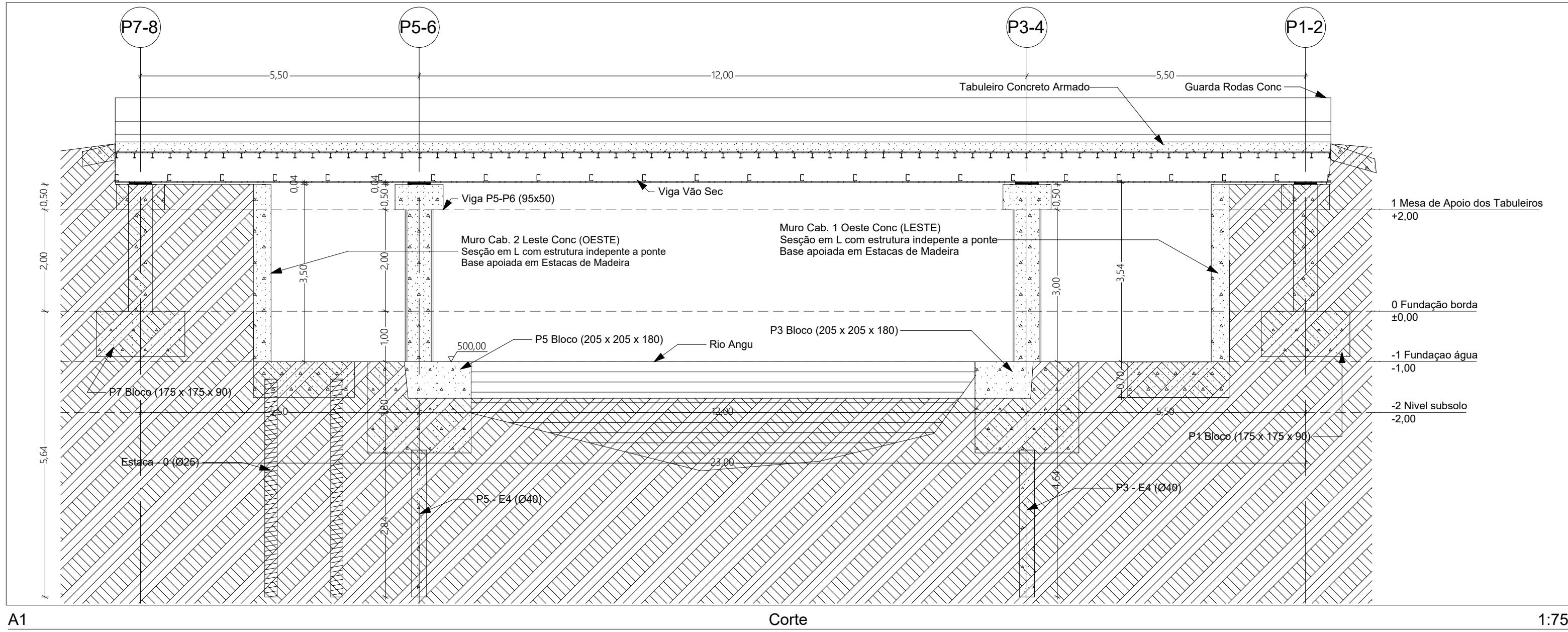
A1 Corte 1:75
