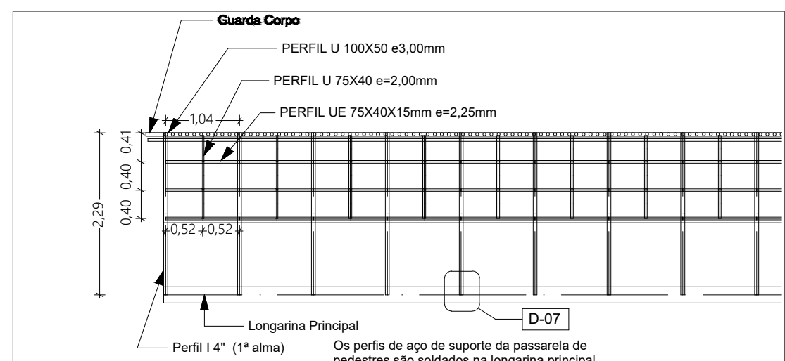
EST-10 Detalhes estrutura da Passarela de Pedestres 1:75
