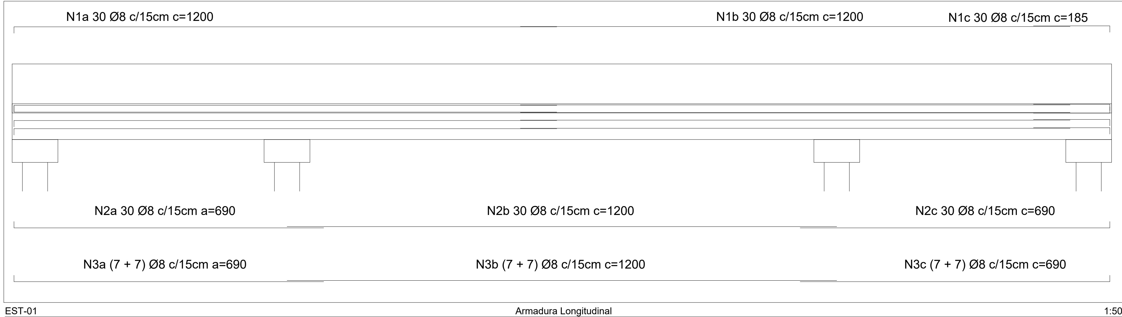
EST-01 Armadura Longitudinal 1:50
