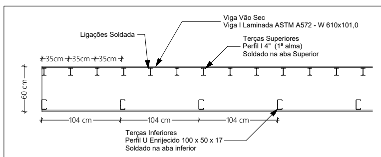
D-05 Distancias entre as Terças 1:50
