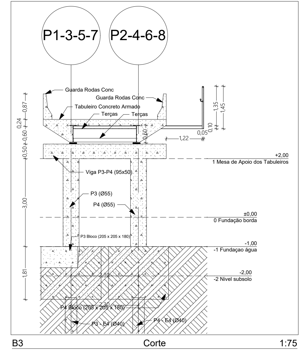
B3 Corte 1:75
