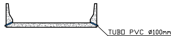
4 DETALHES DA DRENAGEM DO TABULEIRO ESCALA 1:100
