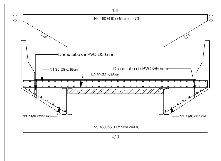
D-02 Seção Tabuleiro Concreto Armado 1:50
