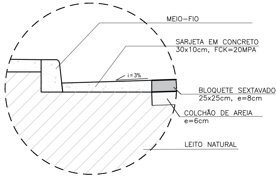
3 DETALHE 01 SEM ESCALA
