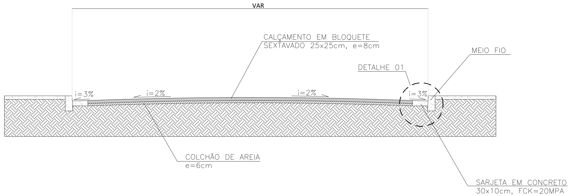
2 CORTE TRANSVERSAL SEM ESCALA
